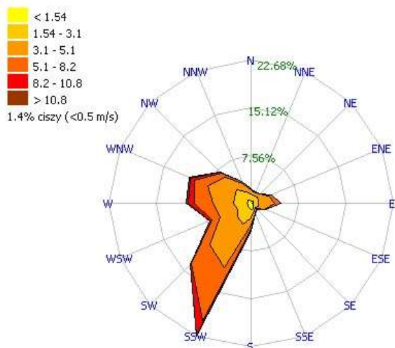
Rysunek 1-10 Rozkład kierunków i prędkości wiatru dla stacji Zgorzelec w 2015 r.
