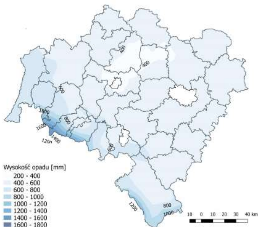
Rysunek 1-17 Przestrenny rozkład rocznych sum opadów atmosferycznych, wyznaczonych przez model WRF/CALMET, w strefie dolnośląskiej, w 2015 r.
